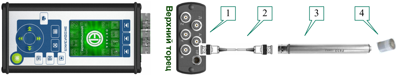
Схема 3. Подключение преполяризованных микрофонов ко входам А, Х, Y, Z
