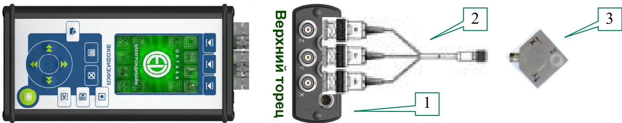
Схема 4. Подключение 3-компонентного датчика ко входам X, Y, Z или X, Y, A
