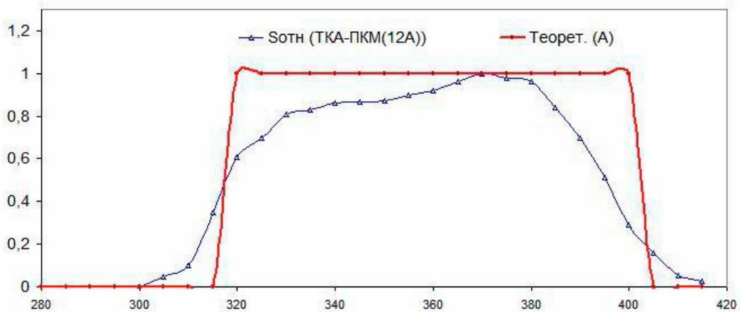
Рис.1 Относительная спектральная чувствительность прибора
