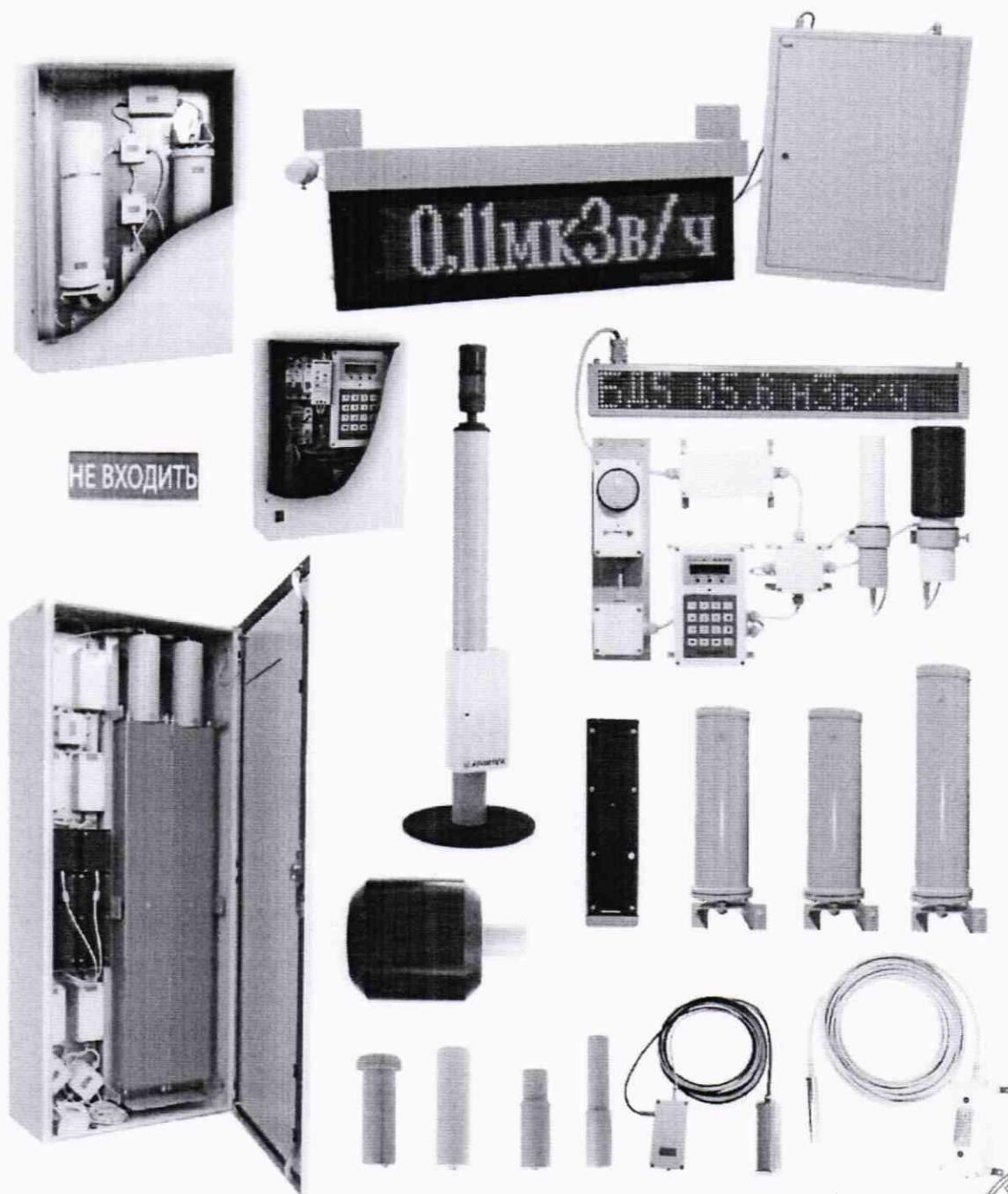
Рисунок 1 – Общий вид измерителя-сигнализатора СРК-АТ2327.
