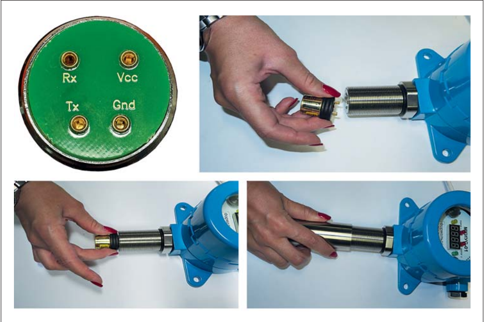
Рис.4. Подключение интеллектуального сенсорного модуля
