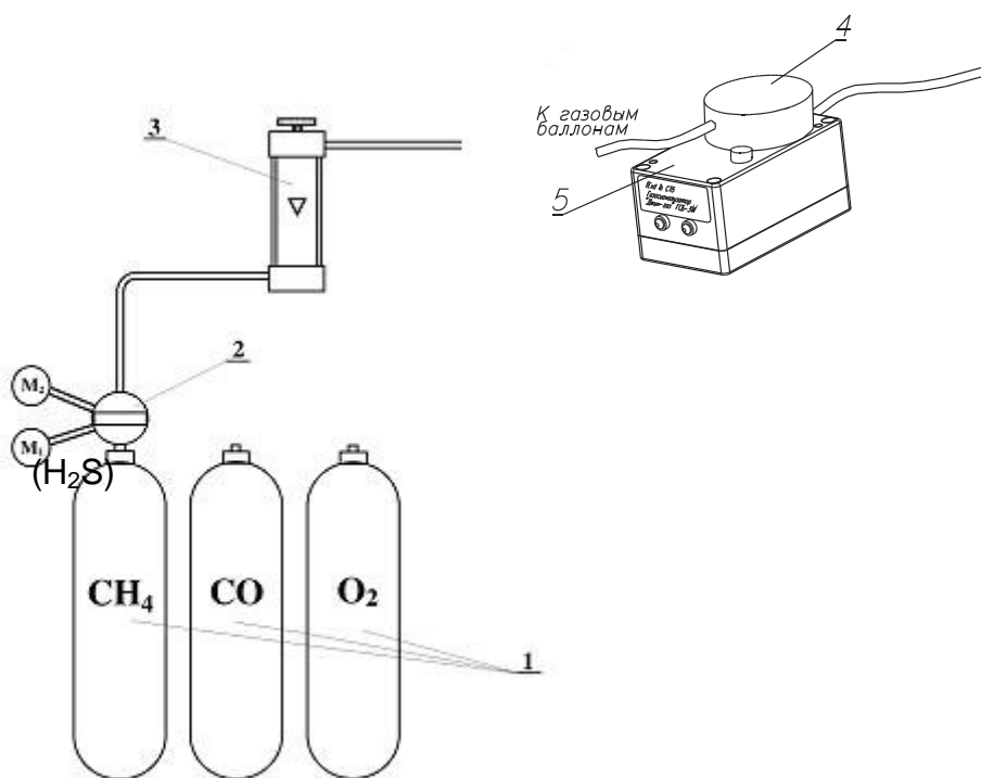
Рисунок 5. Схема стенда для проверки работоспособности газосигнализатора 1 - баллоны с ПГС; 2 - редуктор; 3 - ротаметр; 4 - камера; 5 - измерительный модуль.
