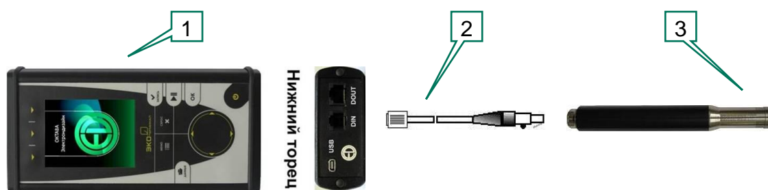
Рис. 1. Подключение ОКТАФОН-110А к ИБ ЭКОФИЗИКА-Д.
