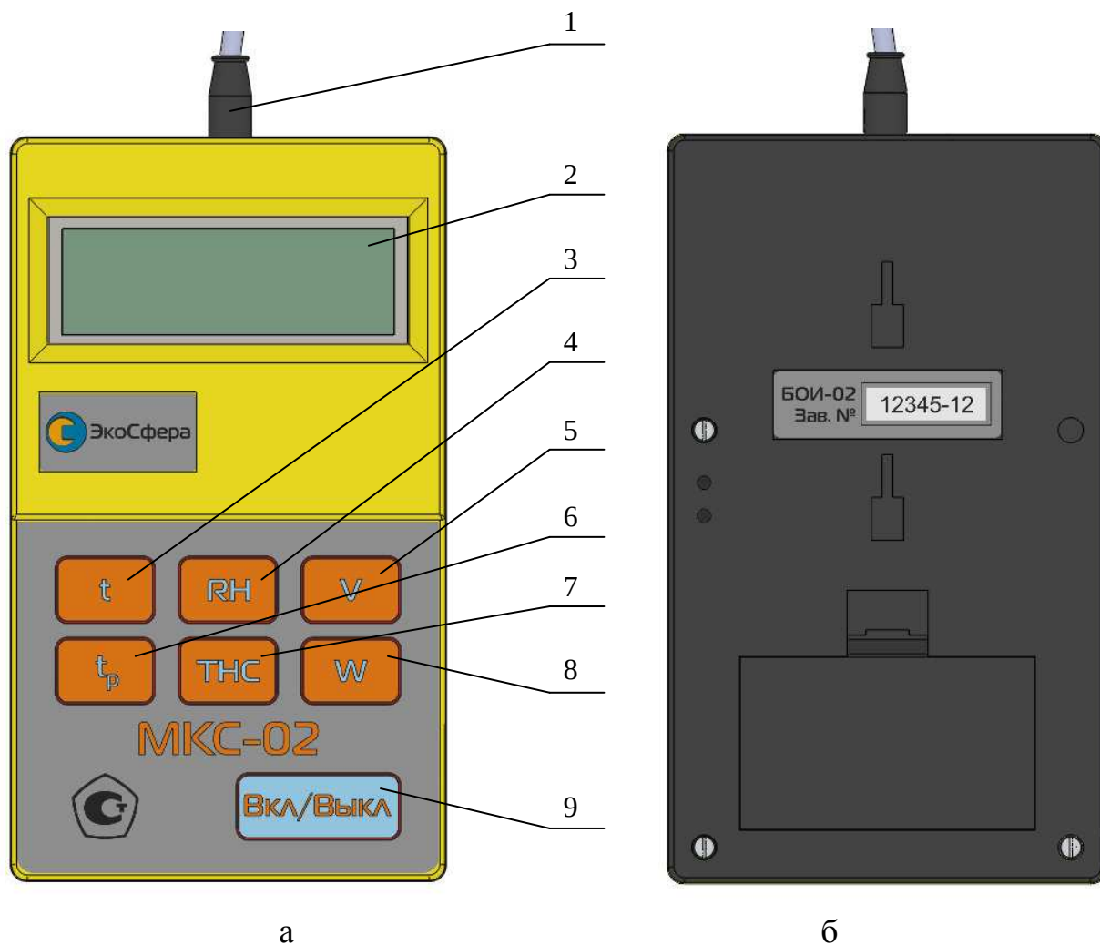
Рис. 1 – Внешний вид блока отображения информации МКС-02 (а - лицевая сторона, б – тыльная сторона)
