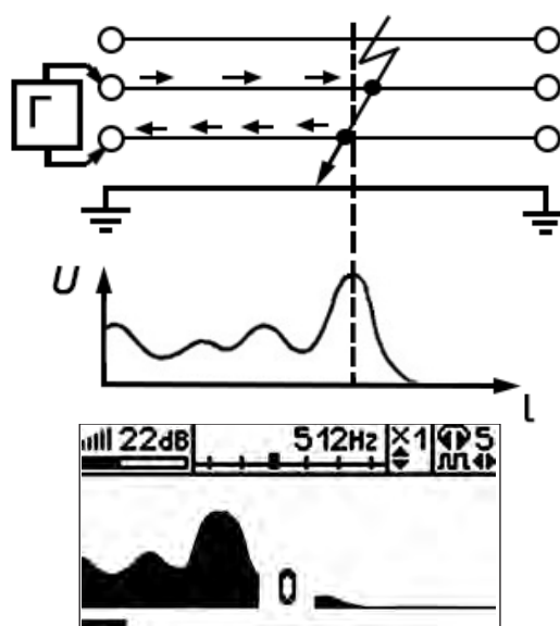
Рис.8.9 КЗ-двухфазное
