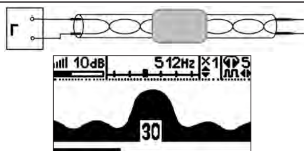
Рис.8.7 Муфта
