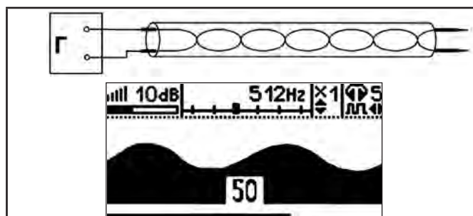
Рис.8.6 Повив
