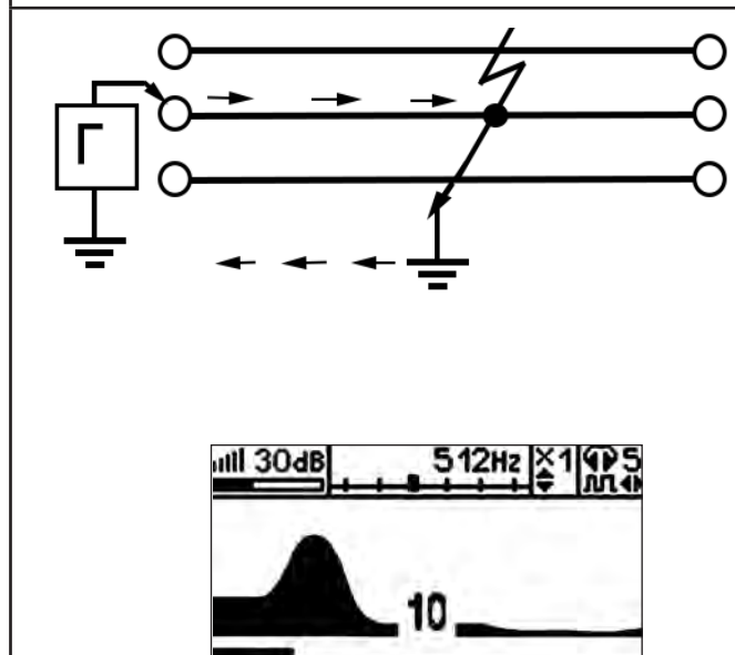
Рис.8.8 КЗ-однофазное
