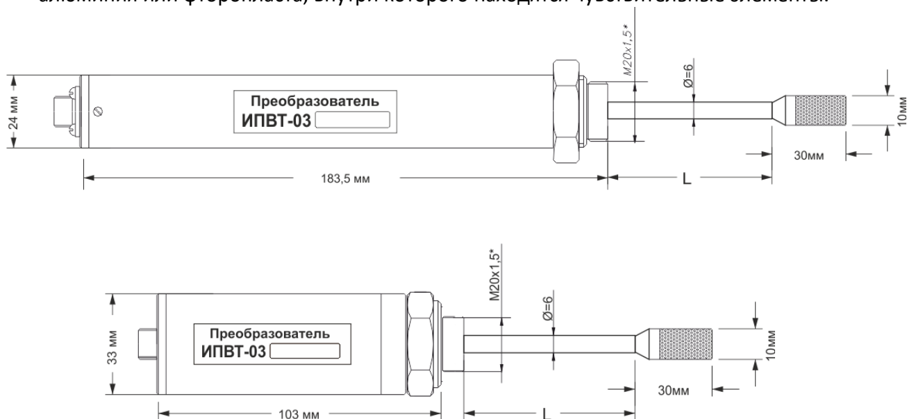
Рисунок В5 Измерительный преобразователь ИПВТ-03-06
