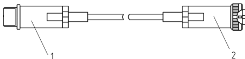
Рисунок 3.4 Кабель-удлинитель для измерительных преобразователей, приведенных в ПРИЛОЖЕНИИ Г в пунктах 1, 4, 6, 7 ;
