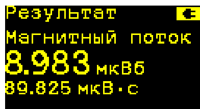
Рисунок 3.9 Результат измерения потокоосцепления
