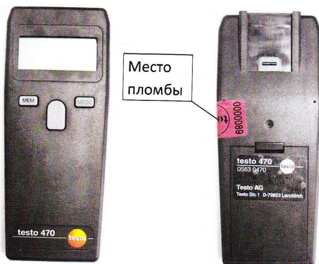
Рисунок 3. Фототахометр электронный Testo-470
