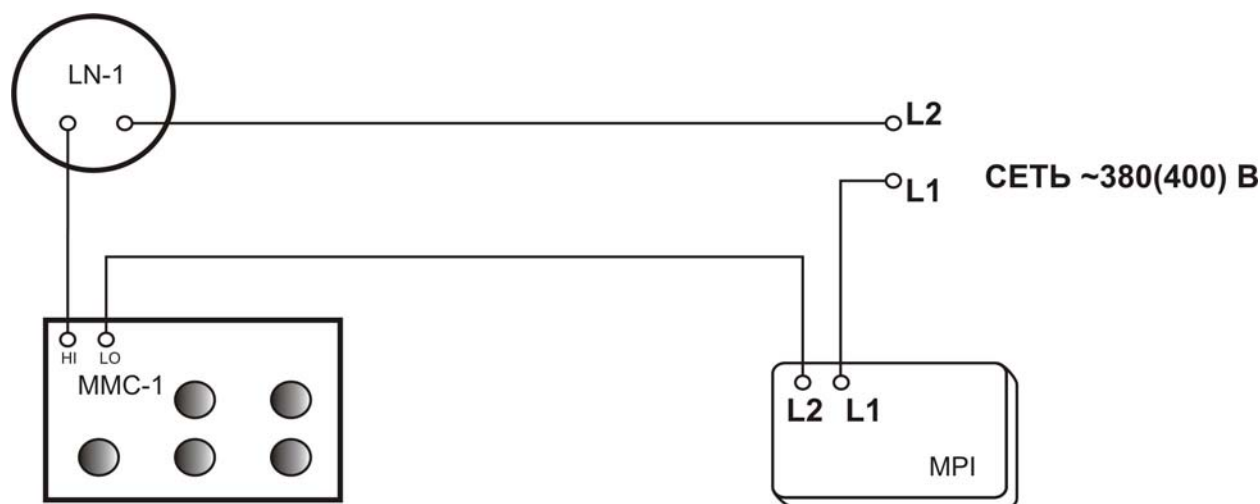
Рисунок 5 - Структурная схема определения абсолютной погрешности измерения полного сопротивления цепи “фаза-фаза”,
