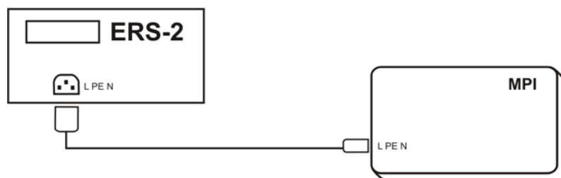
Рисунок 9 – Структурная схема определения абсолютной погрешности измерения времени отключения УЗО,
