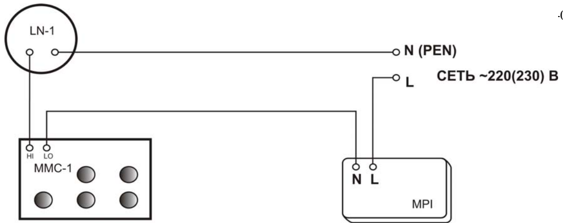
Рисунок 4 - Структурная схема определения абсолютной погрешности измерения полного сопротивления цепи “фаза-нуль”, где МПИ – поверяемый измеритель, ММС-1 – магазин мер сопротивлений петли короткого замыкания; LN-1 – катушка индуктивности силовой цепи эталонная.
