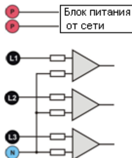
Рис.14 Входы по напряжению и блок питания
