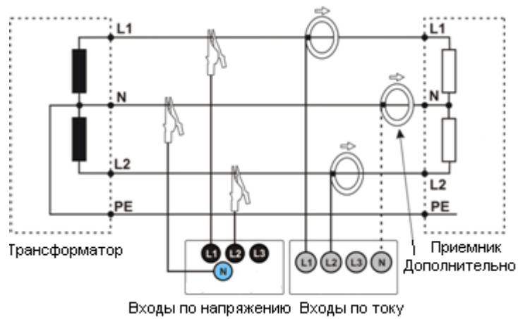
Рис.6 Схема подключения – двухфазная система.
