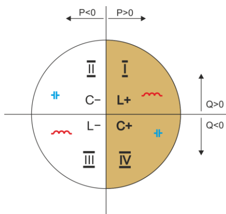
Рис.18 Четырёхквadrатное деление потока мощности и энергии.
