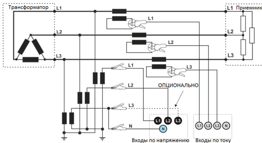
Рис.13 Схема подключения – косвенные измерения в 3-х фазной схеме «треугольник» сети среднего напряжения с измерительными трансформаторами.
