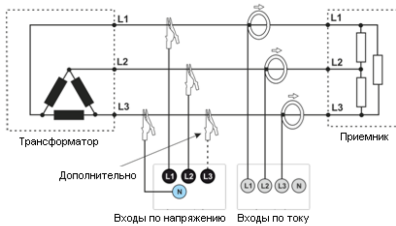
Рис.9 Схема подключения – трёхфазная сеть «треугольник».
