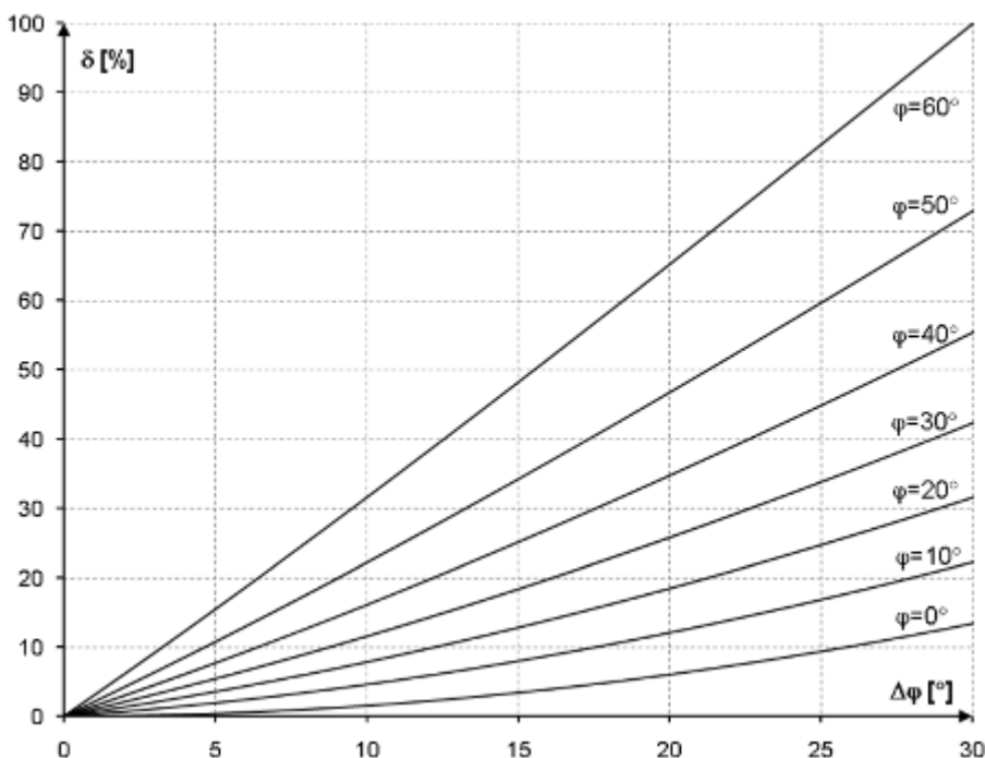
Рис.25 Дополнительная погрешность от ошибки фазы в зависимости от угла сдвига фаз
