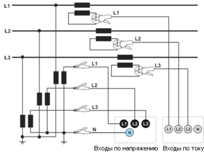
Рис.12 Схема подключения – косвенные измерения в 3-х фазной схеме «звезда» сети среднего напряжения с измерительными трансформаторами.
