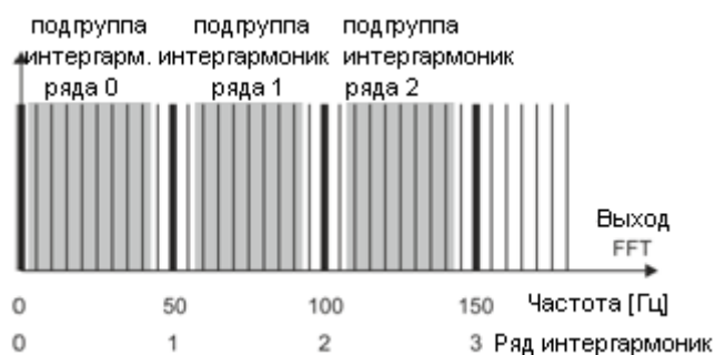
Рис. 42. Определение подгрупп интергармоник (сеть 50 Гц).
