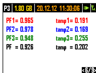
Рис. 10. Экран 6/9 с коэффициентами мощности и \text{tg}\varphi .
