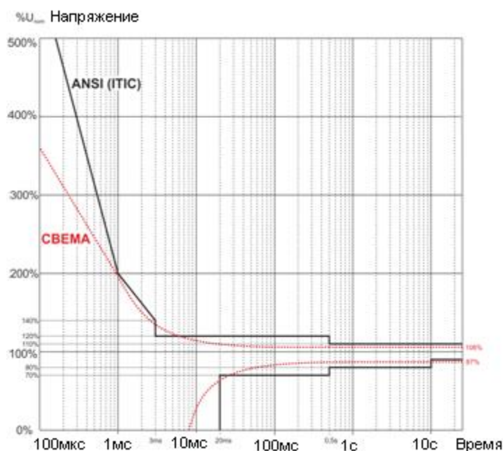
Рис. 53. Линии допустимого диапазона напряжения питания ANSI (ITIC) и СВЕМА.
