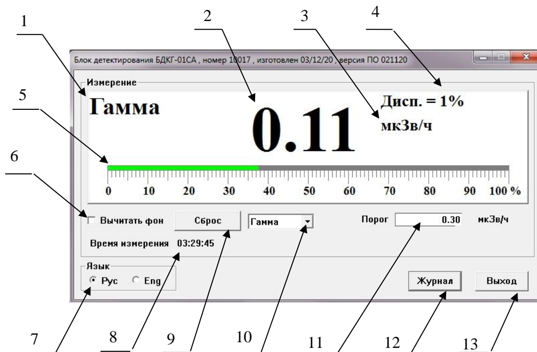
Рис. 9. Окно программы «CONTROL_BD»
